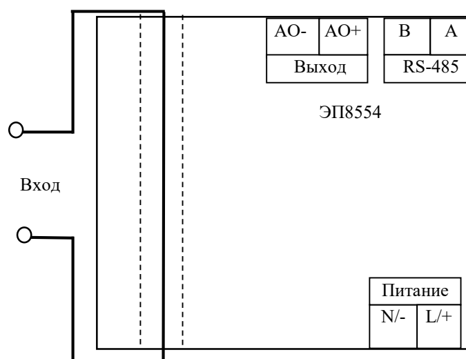
Рисунок Б.9 – Схемы электрическая подключения одноканальных ЭП8554 с номинальными входными сигналами свыше 5 А в корпусе с габаритными размерами 132x81x71 mm
