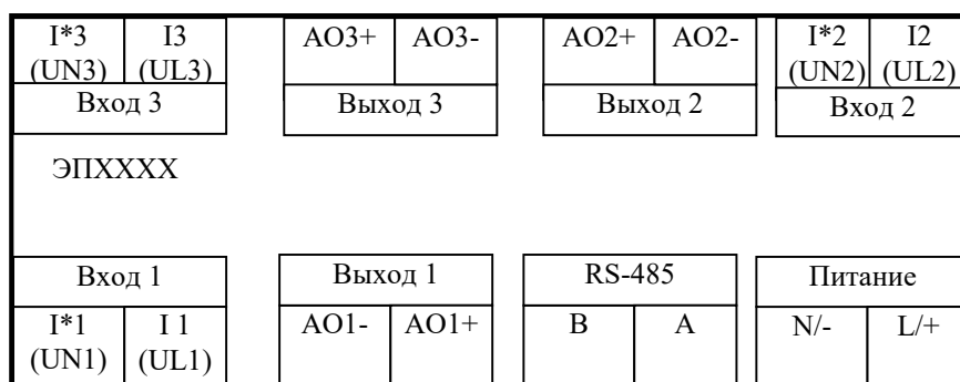
Рисунок Б.5 – Схемы электрическая подключения в трехфазную сеть для измерения линейных напряжений трехканальных ЭП8555 в корпусе с габаритными размерами 110x120x125 mm или 110x120x136 mm
