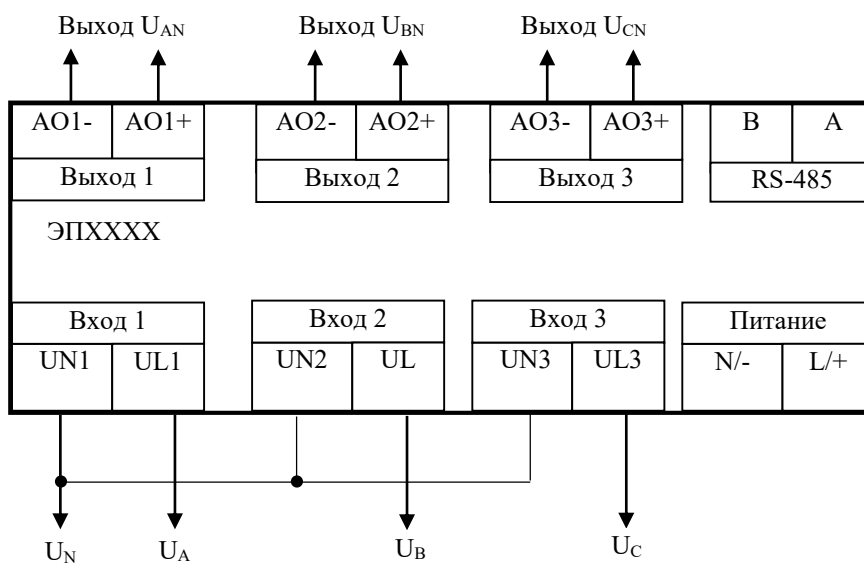
Рисунок Б.4 – Схемы электрическая подключения в трехфазную сеть для измерения фазных напряжений трехканальных ЭП8555 в корпусе с габаритными размерами 110x120x125 mm или 110x120x136 mm
